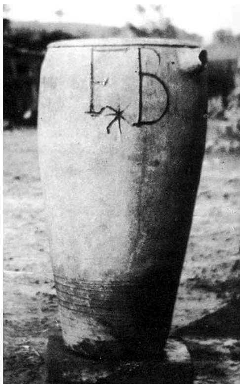
Fig. 4 – “Pignatte” per la distillazione dello zolfo nei cosiddetti “Doppioni” (cf. supra , fig. 2), realizzate a Monte Sasso (Mercato Saraceno) (XVII-XVIII secolo). Esse recano incise, sulle pareti, le sigle dei fabbricanti «A x B» e «F x B»: rispettivamente, Antonio Balducci e Francesco Balducci, entrambi appartenenti ad una famiglia tradizionalmente specializzata in tale produzione (da VEGGIANI 1979).
