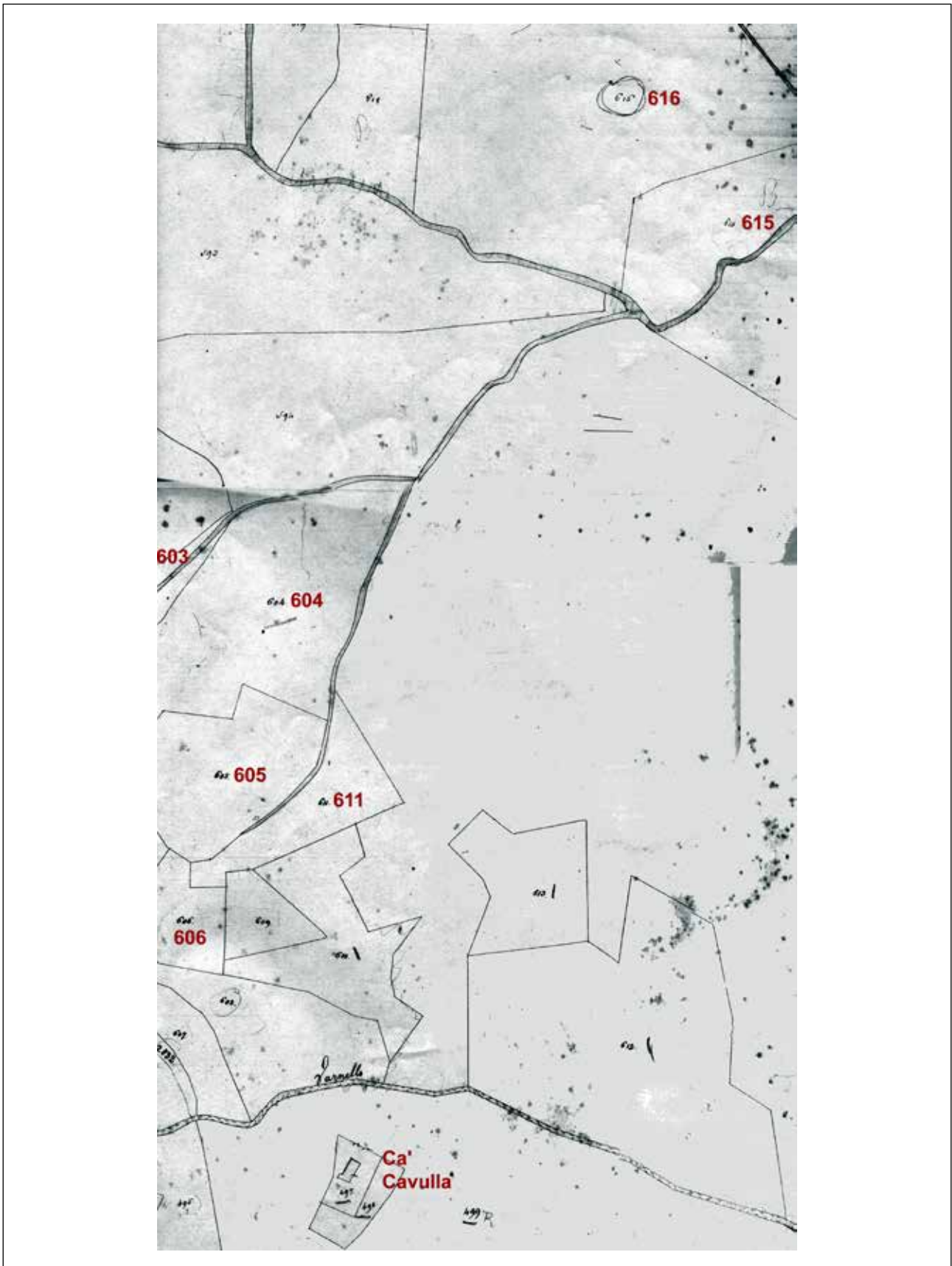
Fig. 5 – ARCHIVIO DI STATO DI RAVENNA, Catasto Gregoriano, Mappa Brisighella, foglio VIII, stralcio. Riproduzione in scala di grigi. Sulla carta, di età napoleonica, sono evidenziati in rosso: Ca' Cavulla; i mappali 603-606 e 611, probabile sede della miniera di zolfo; i mappali 615-616, ubicati nei calanchi delle Argille Azzurre, probabile sede dello stabilimento di raffinazione dello zolfo. Come emerge dalla carta, all'epoca la strada da Brisighella verso Rontana correva a valle di Ca' Cavulla, e non a monte di essa come attestato ai nostri giorni.
