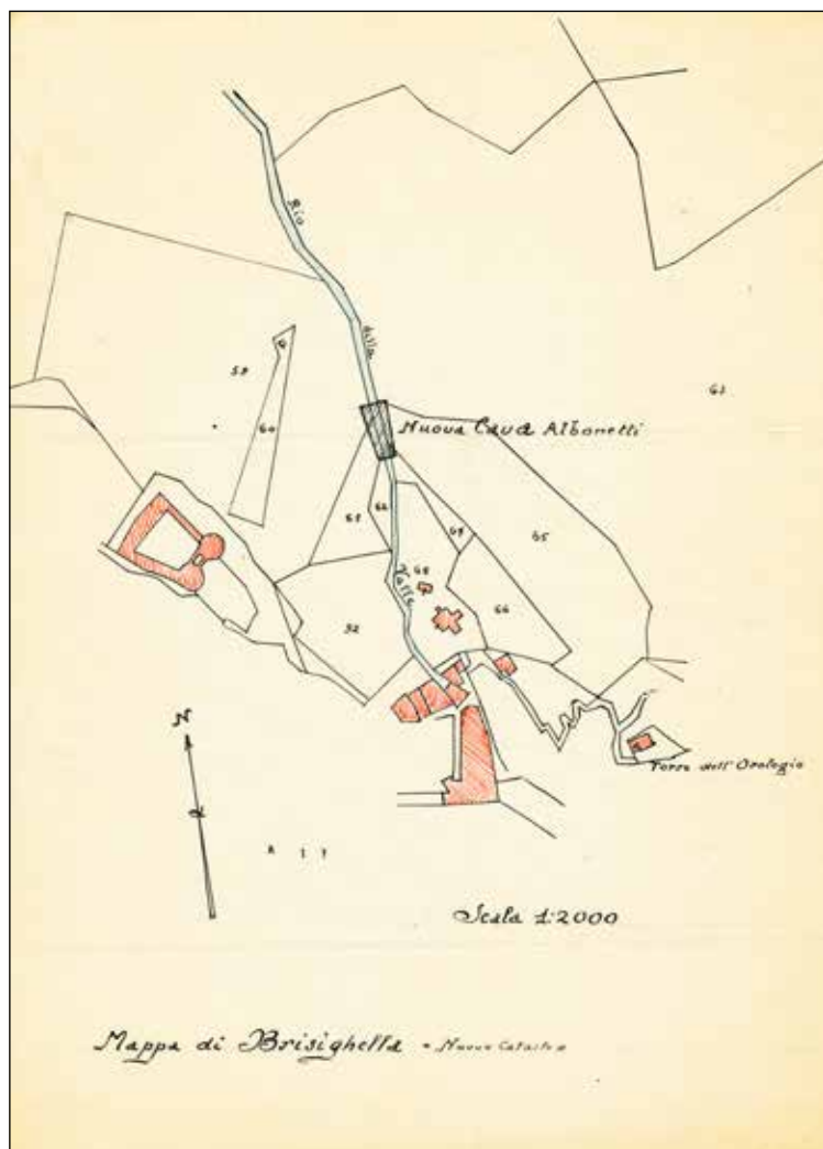
Fig. 25 – Carta di lavoro anonima conservata in ADMB, datata 1927, nella quale è rappresentato un terzo sito estrattivo a conduzione Bassi, da aprirsi in una modesta placca gessosa (di crollo?) ubicata nei pressi del fondo della valle cieca del Rio della Valle, in corrispondenza del corso stesso del Rio. Nella mappa, l'indicazione «Nuova Cava Albonetti» fa riferimento al nome del proprietario del terreno, e non alla conduzione della cava. Scopo di tale nuova apertura era verosimilmente quello di proseguire l'escavazione, bloccata alla base del colle della Rocca in seguito alle frane del 1921 e del 1924. Il nuovo fronte di fatto non diventò mai operativo, poiché il Decreto Prefettizio n. 5665 del 23 aprile 1928, in seguito ad un nuovo imponente crollo, decretò la fine di qualunque lavoro presso i due colli brisighellesi più orientali. La carta appare ricalcata a partire da un foglio catastale, riportando i mappali dei vari fondi; gli edifici sono tratteggiati in rosso, riportando il gruppo di edifici originariamente allineati presso l'imboccatura del tombamento del Rio della Valle, poi abbattuti nel 1939 in seguito a una frana. La precisione della carta di progetto è decisamente superiore rispetto a precedenti rappresentazioni "estemporanee", come ad esempio quella qui pubblicata come fig. 12. Scala originale 1:2000.
