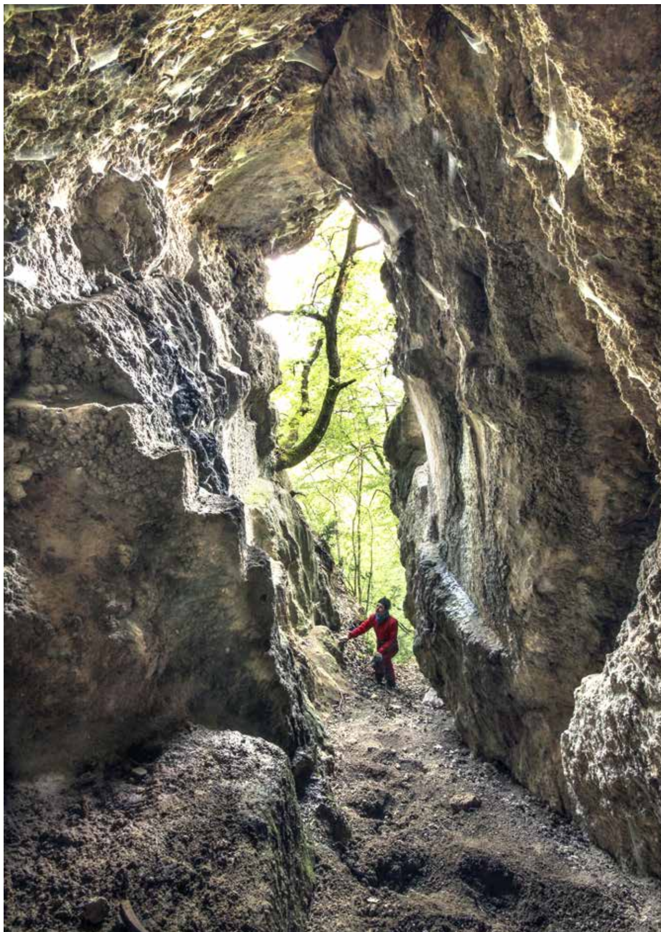
Fig. 24 – La Grotta I “Preistorica” di Castelnuovo. Lungo le pareti sono ben visibili nicchie, mensole e una “scaletta rupestre” ricavate artificialmente, verosimilmente funzionali ad utilizzare la cavità come cantina, ripostiglio o magazzino (foto P. Lucci).
