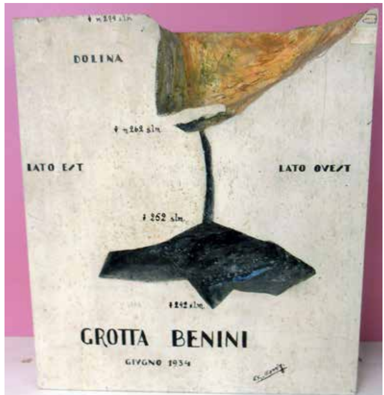
Figg. 10-11 – Plastici realizzati da Giovanni Mornig negli anni Trenta del secolo scorso per la saletta speleologica del Liceo “Torricelli” di Faenza e ora conservati presso il Museo Civico di Scienze Naturali di Faenza. Nella «Grotta Benini» va identificato l’odierno Buco del Noce (foto M. Sami).
