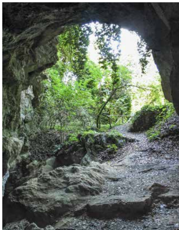
Fig. 4 – La Tanaccia di Brisighella vista dall’interno (foto P. Lucci). Il profilo dell’imboccatura, specie alcune “cornici” aggettanti sulla sinistra dell’immagine, consentono di identificare in tale grotta la cavità ritratta nel 1935 da Pasquale Raggi (fig. 3) per la copertina del volume di G. Bertini Mornig Grotte di Romagna , poi edito postumo (1995), dedicato ai gessi romagnoli.
