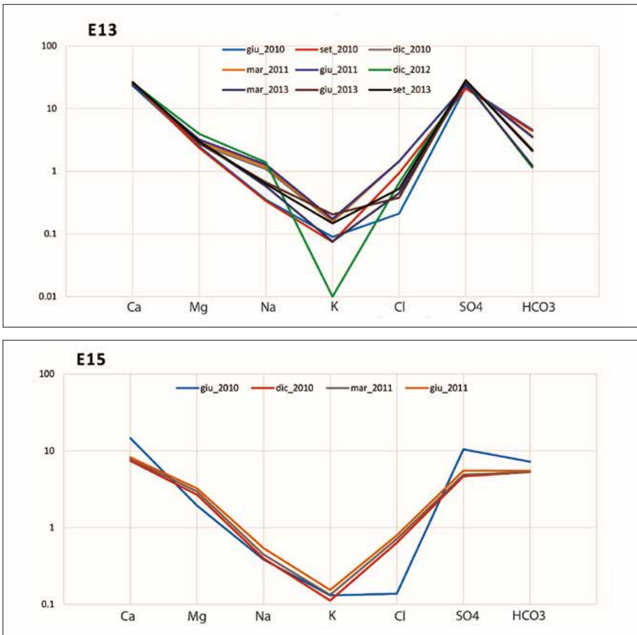
Fig. 4 – Diagrammi di Schoeller per i campioni E13 ed E15. Le concentrazioni dei parametri sono riportate in meq/L.
