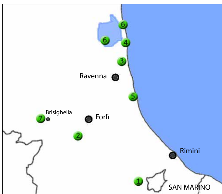
Fig. 11 – Distribuzione di Ononis reclinata in Romagna. Legenda: 1: CHIOSI (1936), Uffogliano (RN), recentemente riconfermata in zona ( http://www.actaplantarum.org/floraitaliae/viewtopic.php?f=40&t=49288&p=314844 ); 2: SEMPRINI (1998), Bertinoro (FC); 3: MONTANARI et alii (2010), Pineta San Vitale (RA); 4: LAZZARI et alii (2012), Foce Reno (RA); 5: Eugenia Bugni (2013), Lido di Classe (RA) ( http://www.actaplantarum.org/floraitaliae/viewtopic.php?f=40&t=49438&p=316122 ); 6: PICCOLI et alii (2014), Valli di Comacchio (FE) e Lido di Spina (FE); 7: Presente studio (2014), Monte Rontana (RA).
