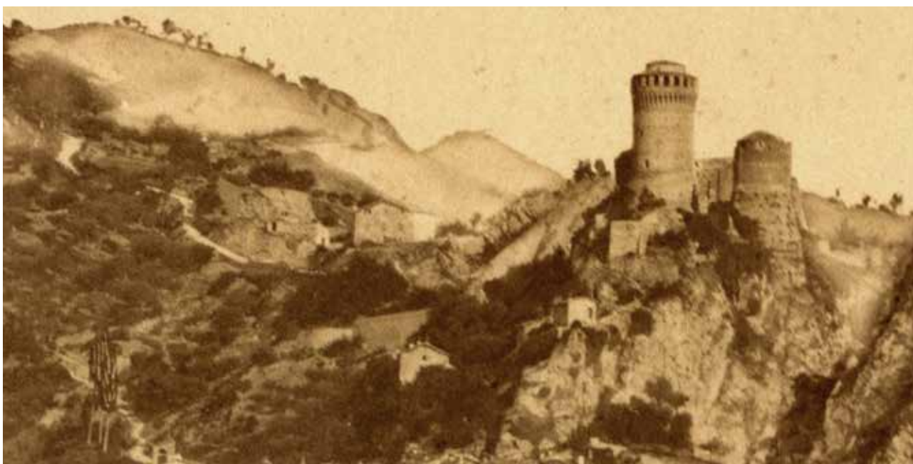
Fig. 44 – Ingrandimento di fig. 43. La scansione dell'originale a 600 dpi permette di cogliere particolari quasi indistinguibili ad occhio nudo, quali una certa continuità dell'affioramento gessoso tra il colle del Monticino e quello della Rocca, ma soprattutto, nella stessa area, un sito estrattivo, con abitazione e fornace annesse, da identificarsi verosimilmente con quello di proprietà Carroli.
