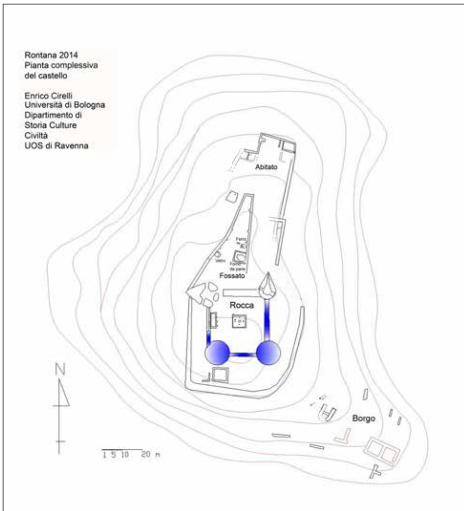
Fig. 3 – Pianta schematica del castello di Rontana, aggiornata alle ultime campagne di scavi (2014). Elaborazione di E. Cirelli.
