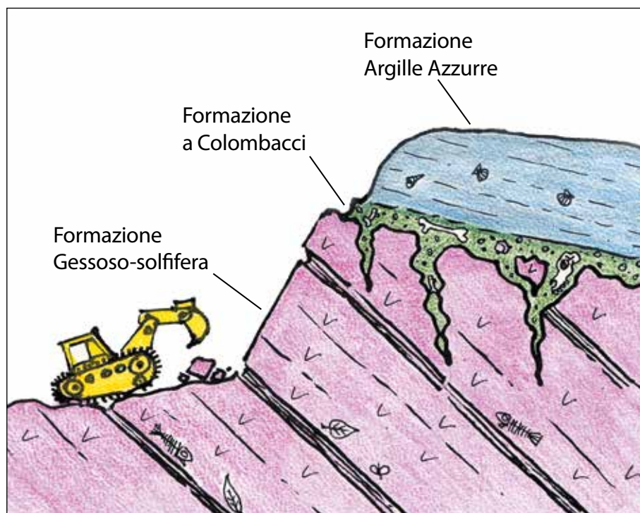
Fig. 2 – Sezione geologica della cava del Monticino (modificato da MARABINI, VAI 1989).
