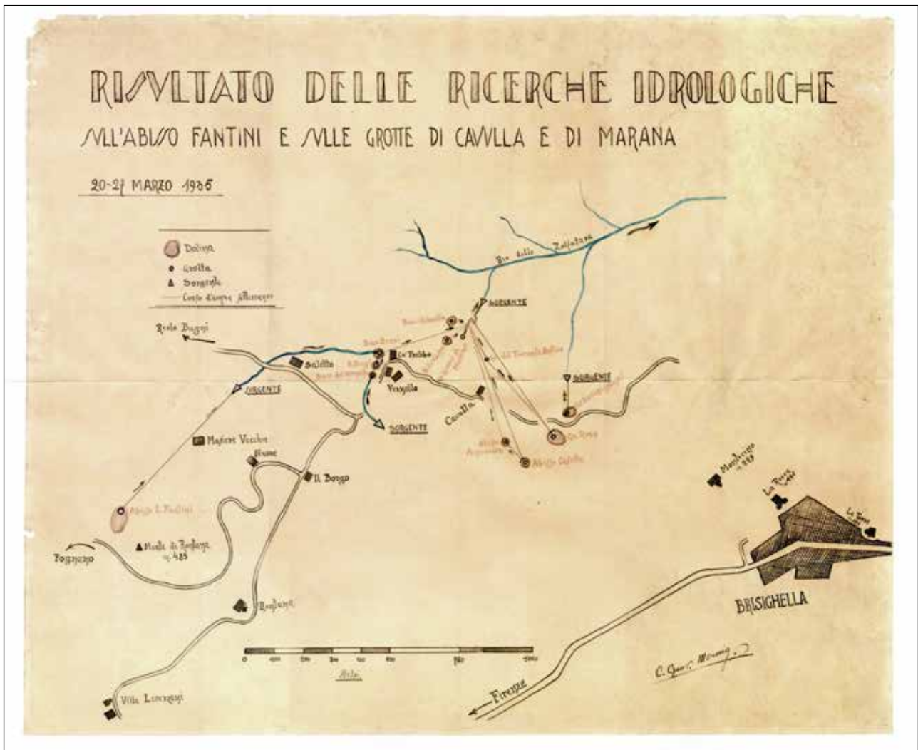
Fig. 8 – Carta idrologica di parte dei Gessi di Brisighella e di Ronzana, disegnata da Giovanni Mornig nel 1935 (da MORNIG 1995). Il corso d’acqua che scorre nel fondo dell’Abisso Fantini non torna a giorno tramite una risorgente ubicata a nord delle “Masere” come indicato nella carta, bensì circa 1,5 chilometri a nord-ovest, tramite la Risorgente del Rio Cavinale. Mornig fa inoltre convergere le acque delle Grotte Biagi e Brusini [sic] con quelle dell’Abisso Acquaviva e della Grotta Rosa Saviotti in un’unica risorgente. In verità si tratta di due distinte risorgenti, separate da poche decine di metri. Infine, le acque del Buco del Noce dovrebbero, secondo Mornig, tornare a giorno poche decine di metri a nord della cavità tramite una risorgente che però non è mai stata individuata.
