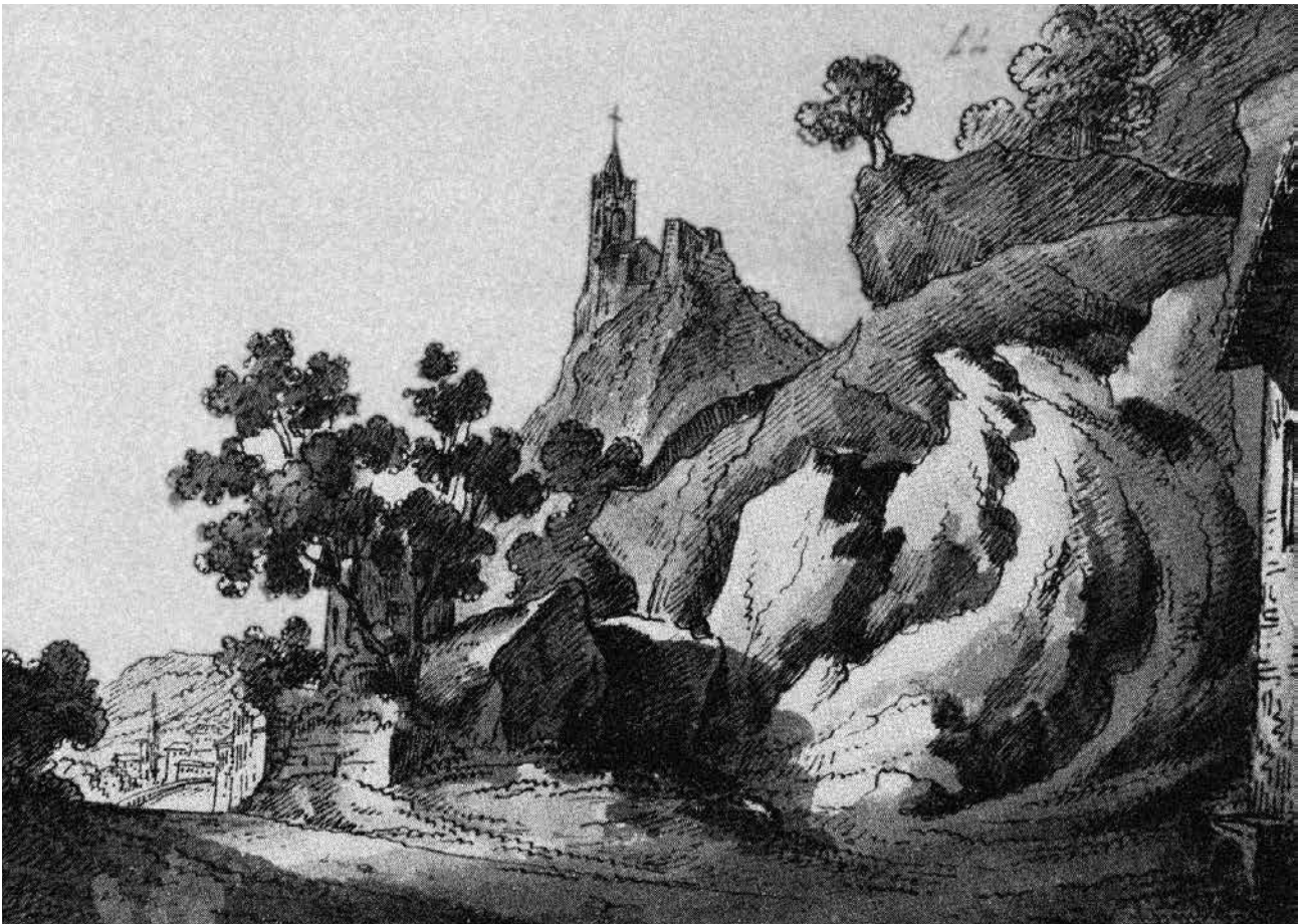
Fig. 4 – Le pendici orientali del colle della Torre dell’Orologio in un disegno dell’artista faentino Romolo Liverani risalente alla metà del XIX secolo circa (da Aa.Vv. 1974). Le singolari morfologie gessose visibili in primo piano possono forse essere riferibili all’azione di una cava. La torre qui ritratta da Liverani è il fortilizio nella sua configurazione precedente alla sua demolizione e successiva ricostruzione (1850) nelle forme neo-gotiche visibili attualmente.
