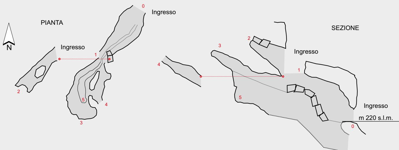
Speleo GAM Mezzano (RA) GROTTA PRESSO CA' LA VALLE ER RA 463 Rilievo (2014): M. Ercolani, P. Lucci, B. Sansavini.
